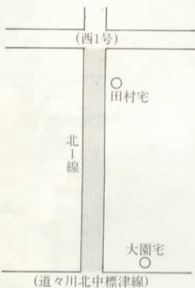
川北北1線地区工事 延長 552 m
