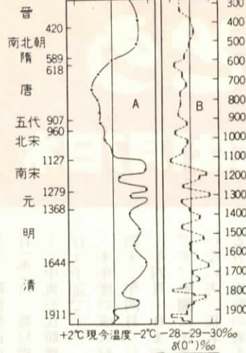
中国(A)及びグリーンランド(B)の気候変動グラフ (竺可楨, 1972による)
