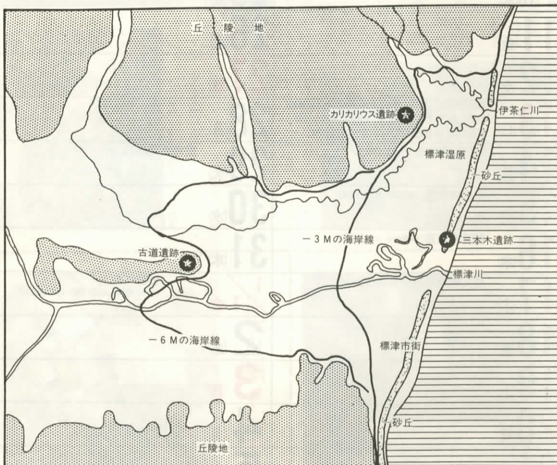
図-3 標津川周辺の縄文海進
