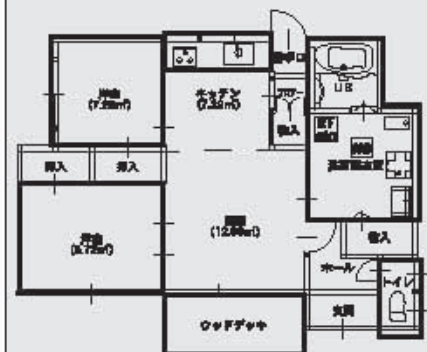
古多量住宅の平面図
