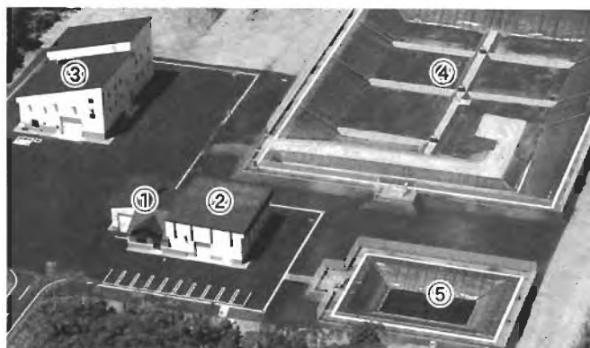
①管理室・計量施設 ②浸出水処理施設 ③前処理破碎施設 ④埋立処分地 ⑤浸出水調整池
