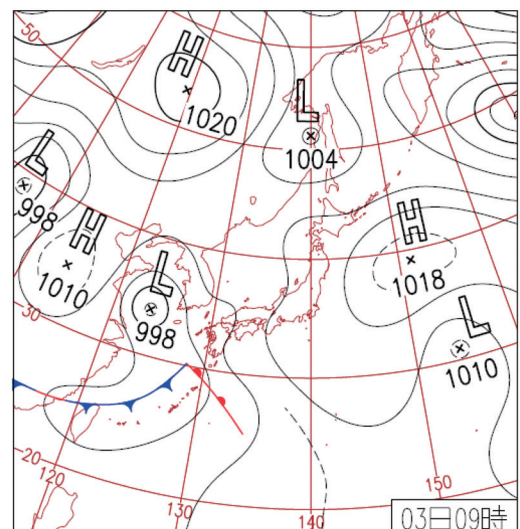
平成26年6月3日9時の気圧配置
