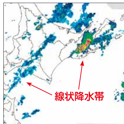
平成27年8月10日20時のレーダーエコー 釧路地方から本町周辺にかけ、活発な線状の 降水域（線状降水帯）が分布する。この他下 北半島からオホーツク管内にかけても線状の 雲が認められる。（図は気象庁提供） ※この日の標津の1時間雨量は 観測史上最大を記録
