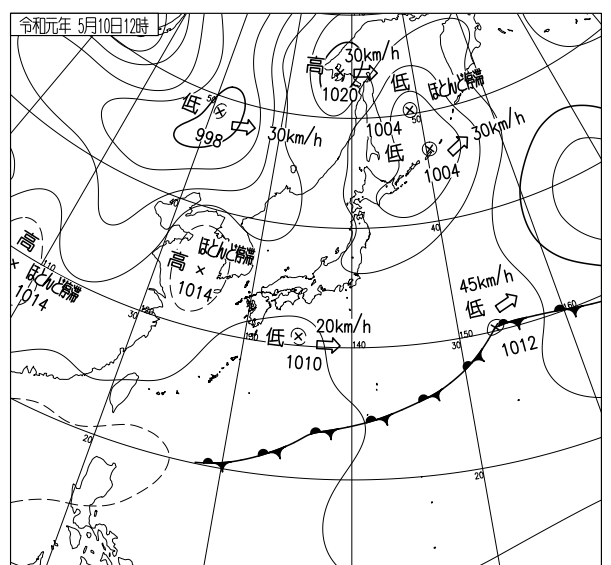
令和元年5月10日12時の地表天気図 この日午前中は晴れていたが、昼過ぎからは雨となった。 (図は気象庁の速報天気図)
