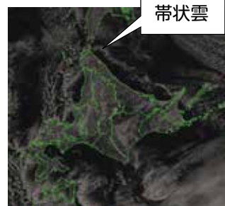
H28.1.30の発生例 (気象庁による衛星可視画像)
