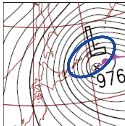
平成26年2月17日9時 このように千島列島付近に 低気圧がある場合は 暴風雪 ※気象庁の図に加筆
