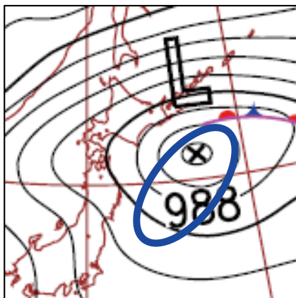
平成22年1月6日9時 このように釧路・根室沖に 低気圧がある場合は 湿った大雪 ※気象庁の図に加筆
