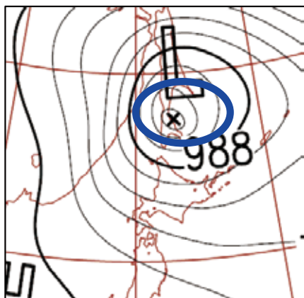
平成24年12月7日9時 このようにサハリン付近に 低気圧がある場合は 晴れ ※気象庁の図に加筆
